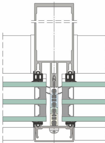
PRZEKRÓJ PRZEZ SŁUP FA 50N
